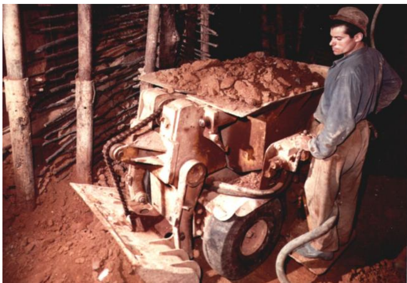
96. ábra Cano-310 rakodógép (MAM)
