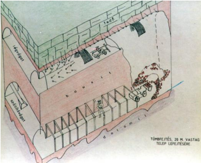
119. ábra. Hazafelé haladó, talpjövesztéses, főtelfüggesztéses tömbfejtési mód vázlatja
