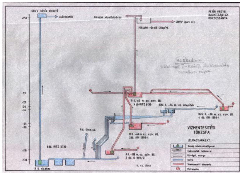
105. ábra Rákhegy II. Vízbánya. Vízkiemelés vonalas rajza (MAM)
