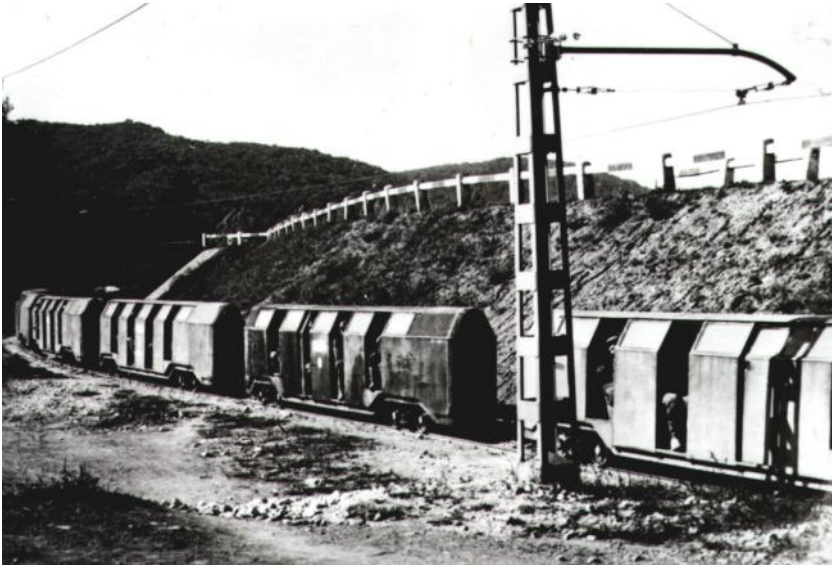
98. ábra Népeskocsis személyszállítás (MAM)
